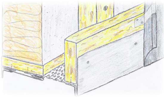
herkömmliche Bauart
